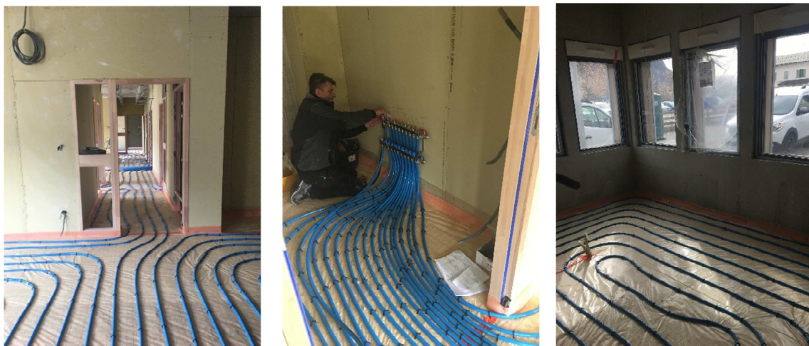
La pose de 800m de tuyaux pour le chauffage au sol.
